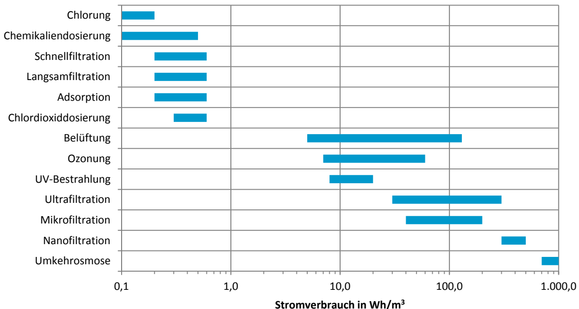
Abbildung 4. Spezifische Stromverbräuche bei Wasseraufbereitungs- bzw. Desinfektionsverfahren (Bundesamt für Energie und SVGW, 2004; DVGW, 2010; Mutschmann & Stimmelmayr, 2011)
