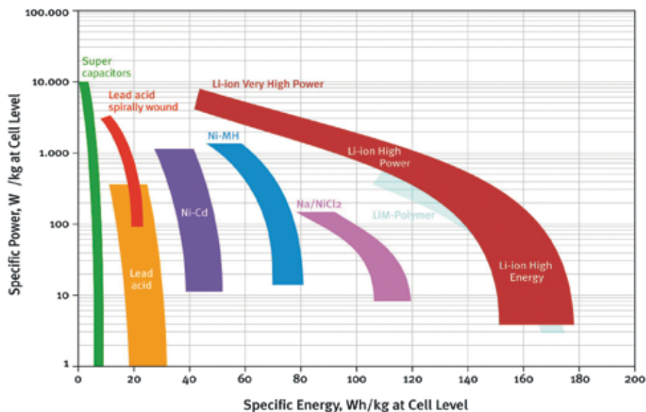
Spezifische Leistungs- und Energiedichten unterschiedlicher Batterietypen. Quelle: Saft Batteries, Johnson Controls, 2007, wiedergegeben in BMLFUW, 2008
